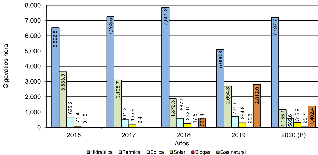
GENERACIÓN BRUTA DE ELECTRICIDAD EN LA REPÚBLICA: AÑOS 2016-20
