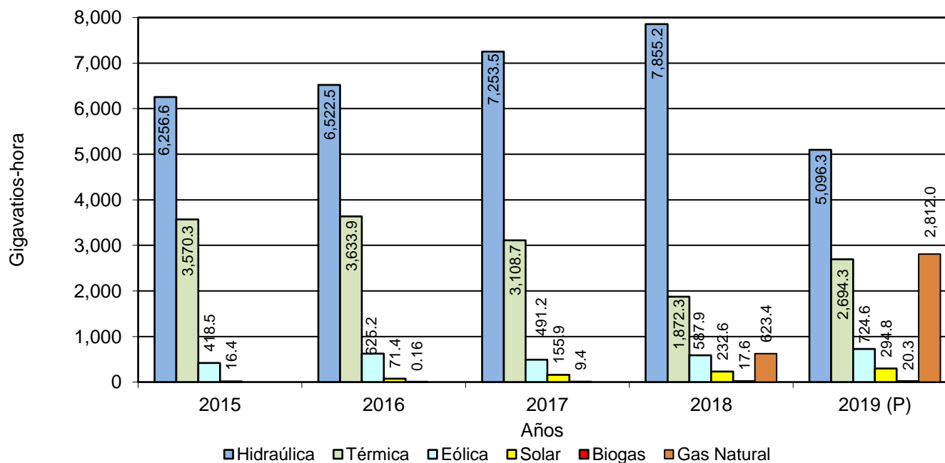
GENERACIÓN BRUTA DE ELECTRICIDAD EN LA REPÚBLICA: AÑOS 2015-19
