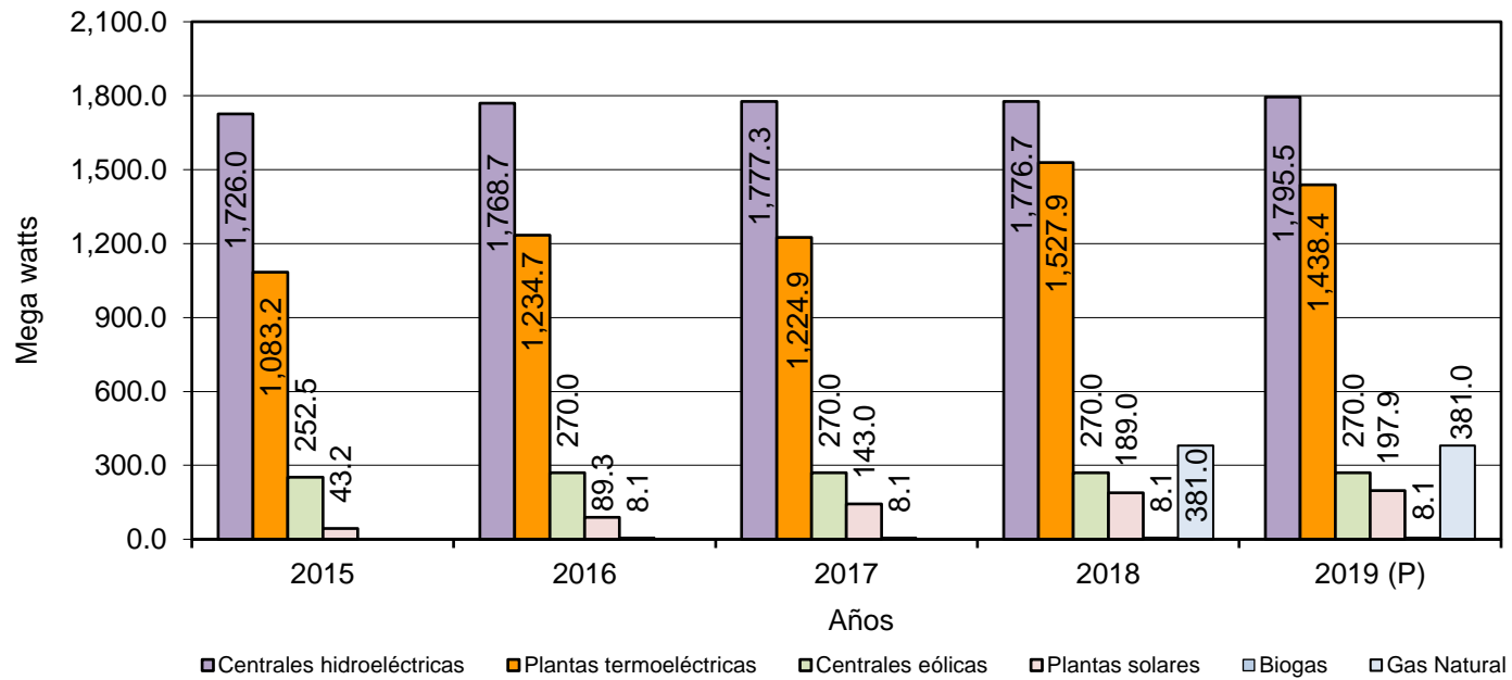
CAPACIDAD INSTALADA DE GENERACIÓN ELÉCTRICA EN LA REPÚBLICA: AÑOS 2015-19
