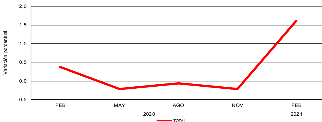
EVOLUCIÓN TRIMESTRAL DEL ÍNDICE DE PRECIOS DE COMERCIO MAYORISTA: FEBRERO DE 2020-FEBRERO DE 2021
